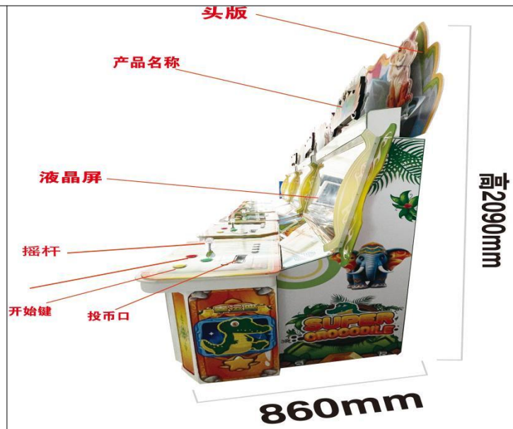
设备外观右侧面照片及说明
